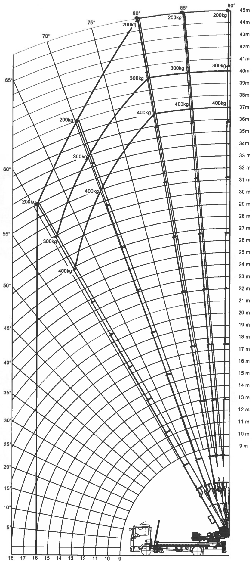
Bigmover 45-6,5
